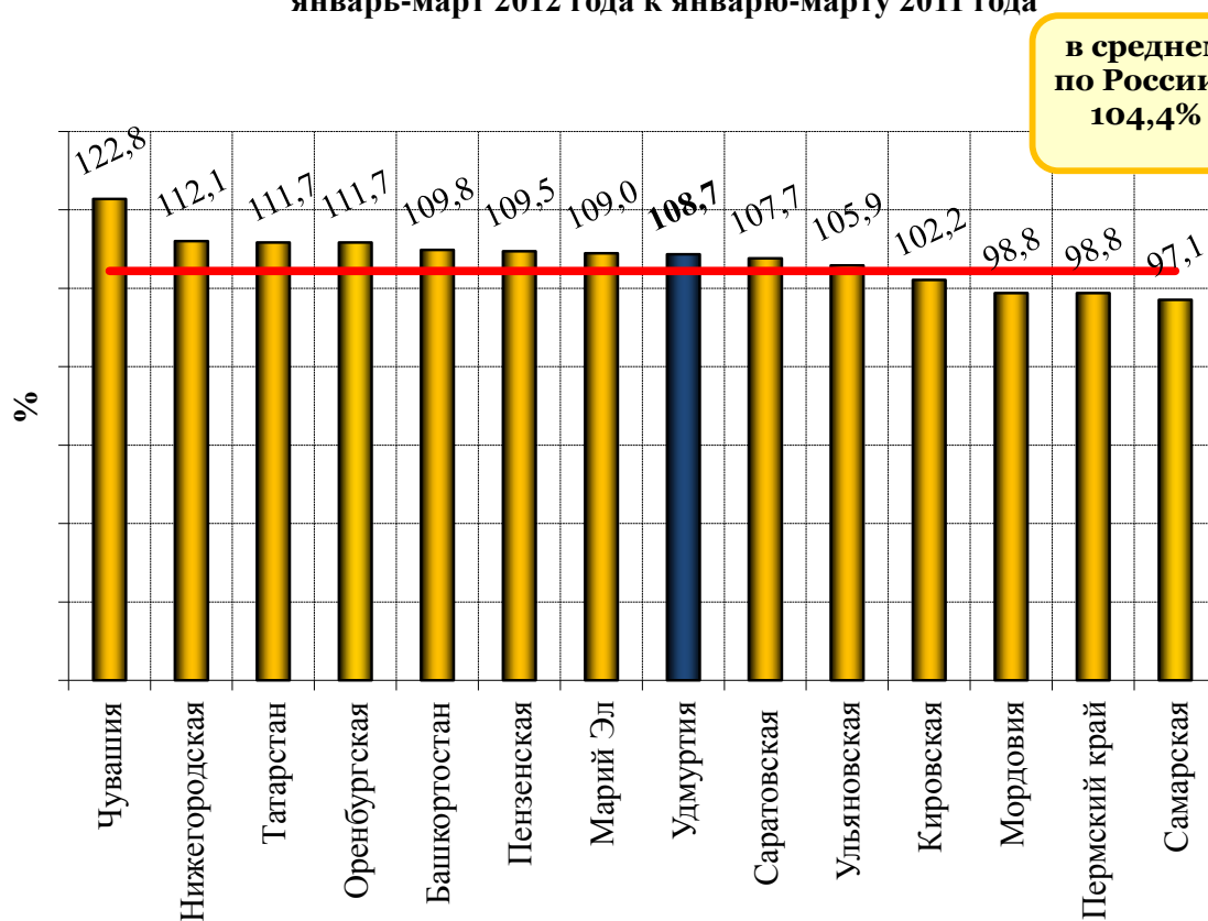
Индекс производства по виду деятельности "Обрабатывающие производства" январь-март 2012 года к январю-марту 2011 года
